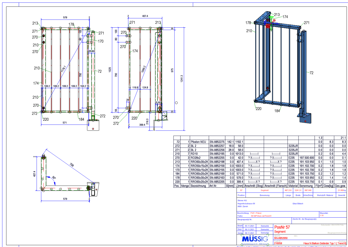
Slika 38: Radionički nacrti Pozicija 57 [11]
