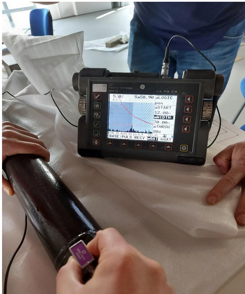
Slika 4. Ultrazvučna kontrola
