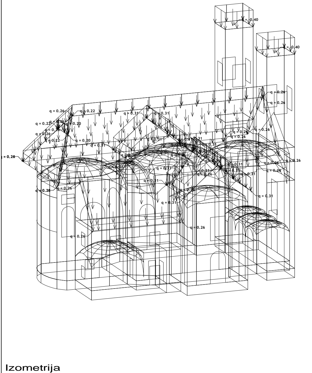
Slika 4.11. Izometrija – Opterećenje 3 – s/2
