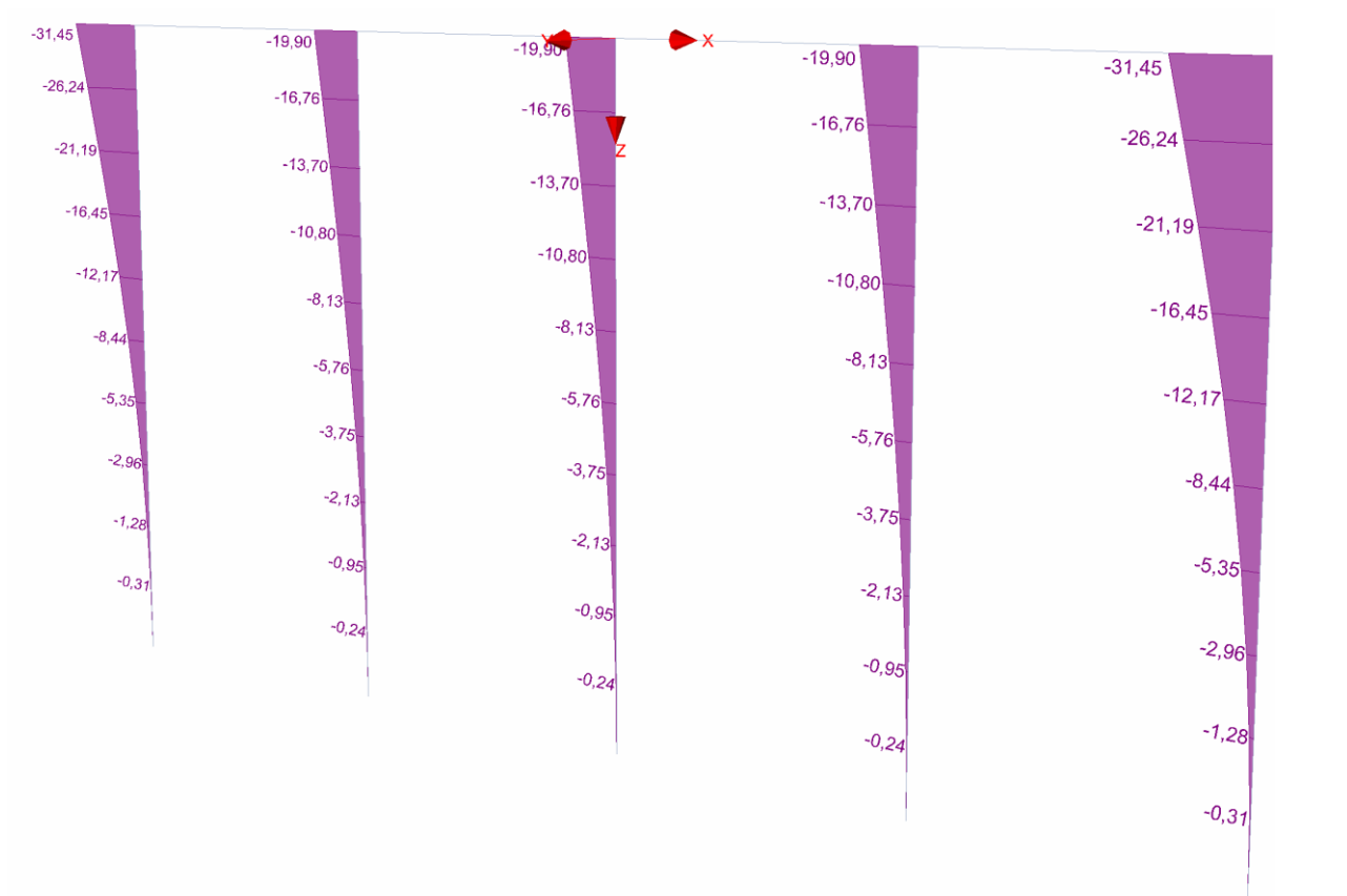
Slika 4.35. Moment Y
