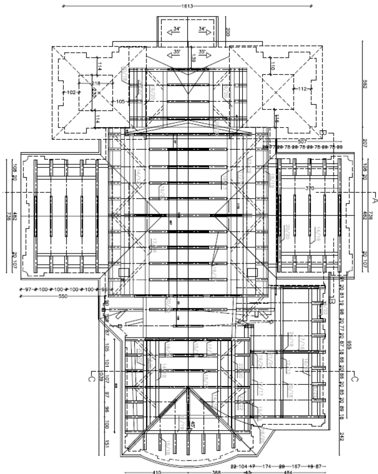
TLOCRT KROVIŠTA M:1:50
