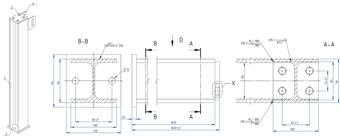
Slika 5.27 Nacrt stupa
