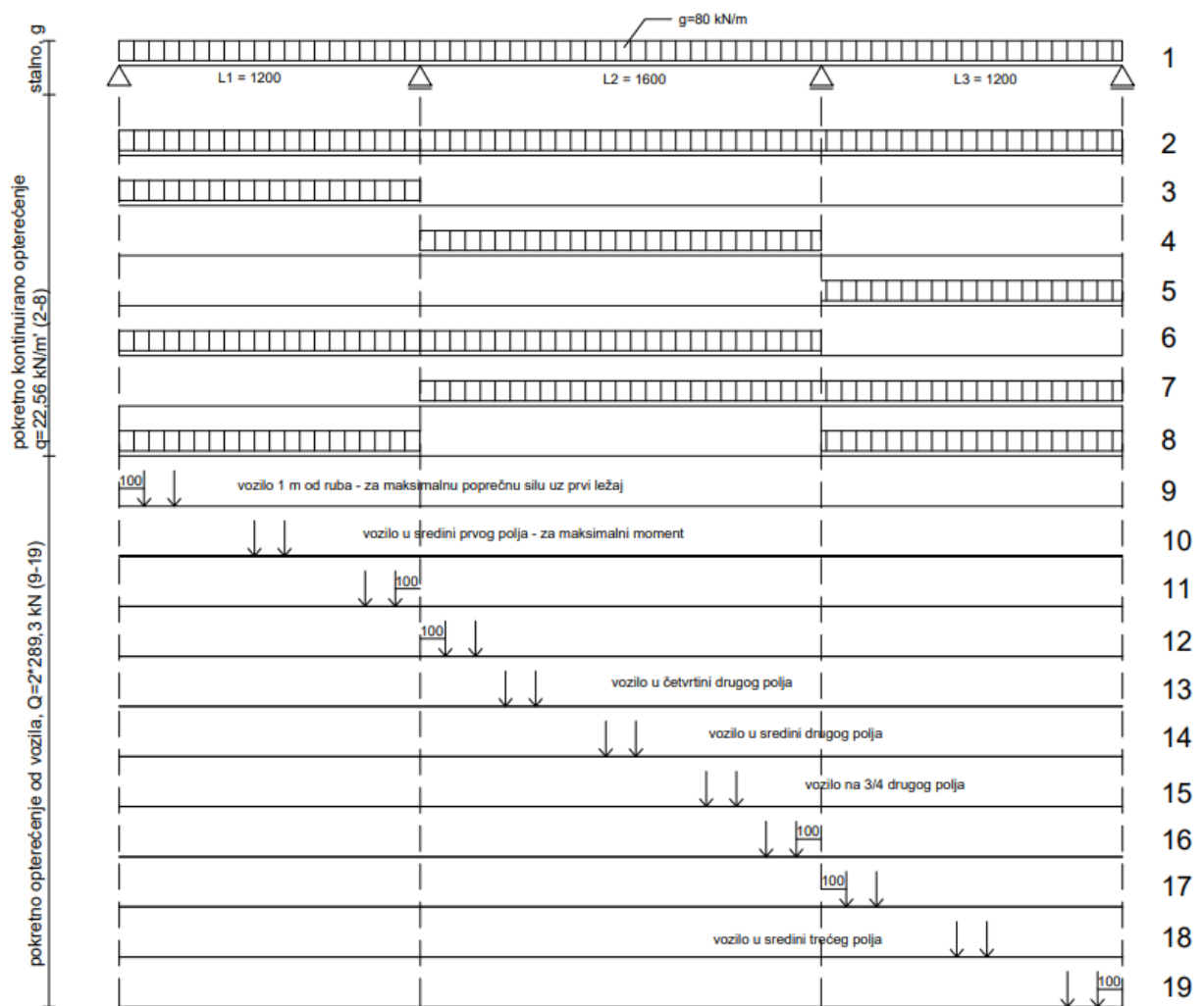
Slika 3.8. Shema slučajeva opterećenja
