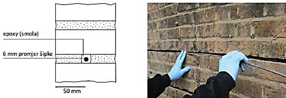
Slika 6.7 - Postavljanje čeličnih šipka [Izvor: 15]
