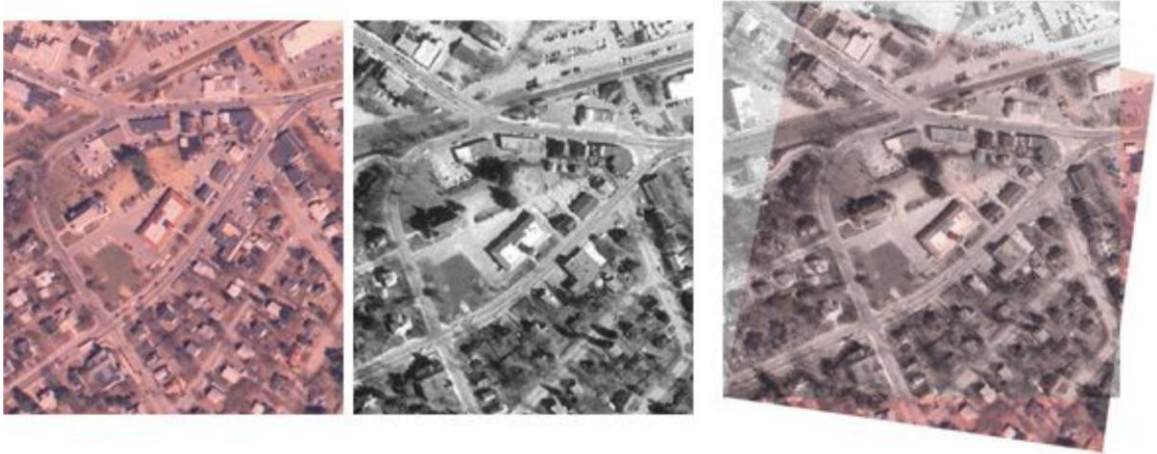
Slika 11: Registracija slike
