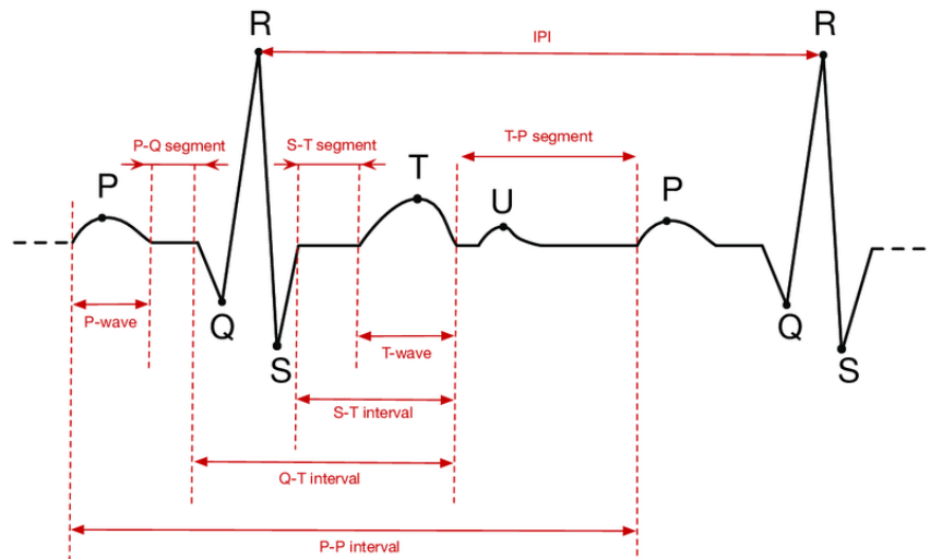
Slika 2.3.1. Elektrokardiogram
