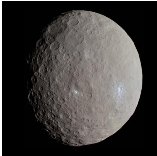
Slika 4 - Ceres [7]
