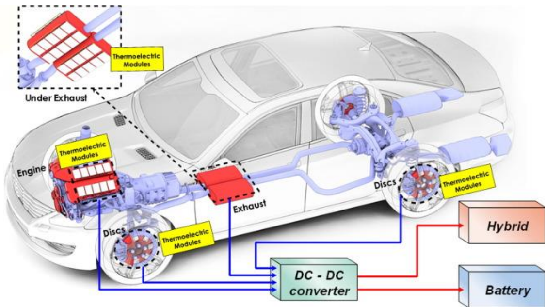
Slika 3.7 Prikaz sustava za recikliranje otpadne topline u automobilima [28]
