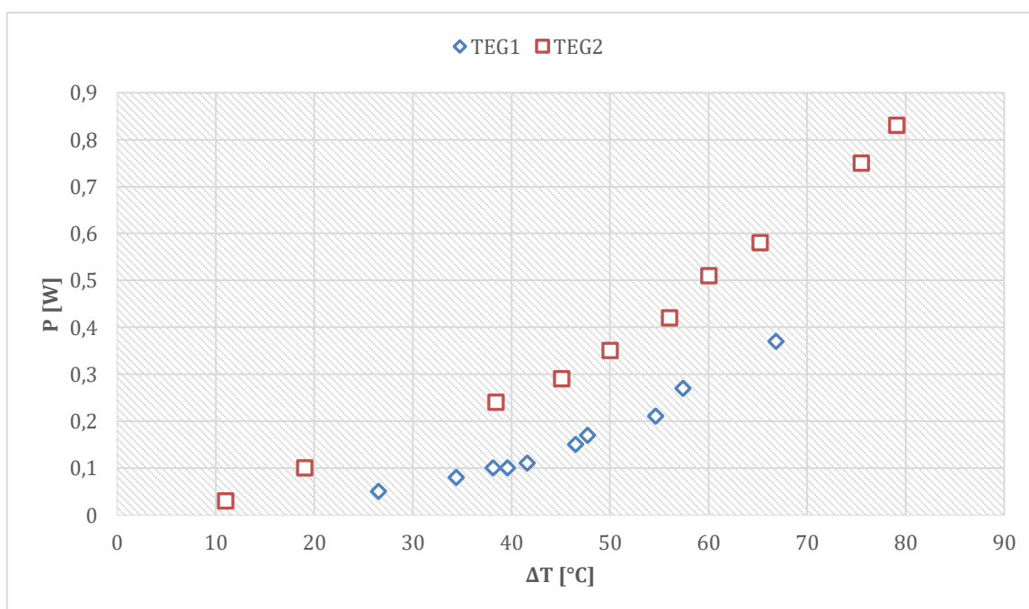
Slika 4.19 Snage termogeneratora TEG1 i TEG2 uz vanjski otpor od 20\Omega
