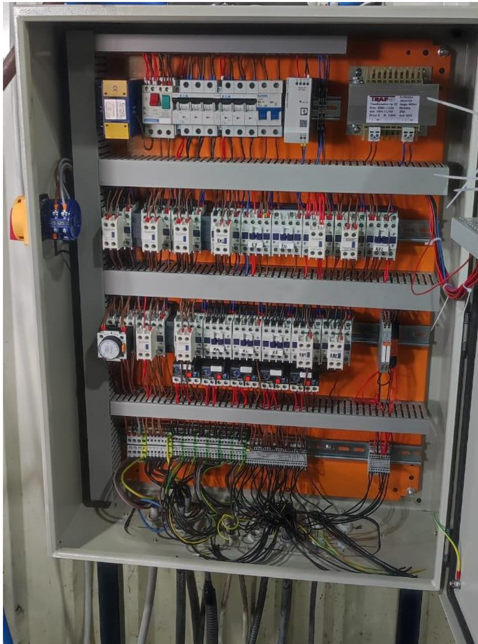
Slika 4.7. Prikaz spoja glavnog i pomoćnog strujnog kruga
