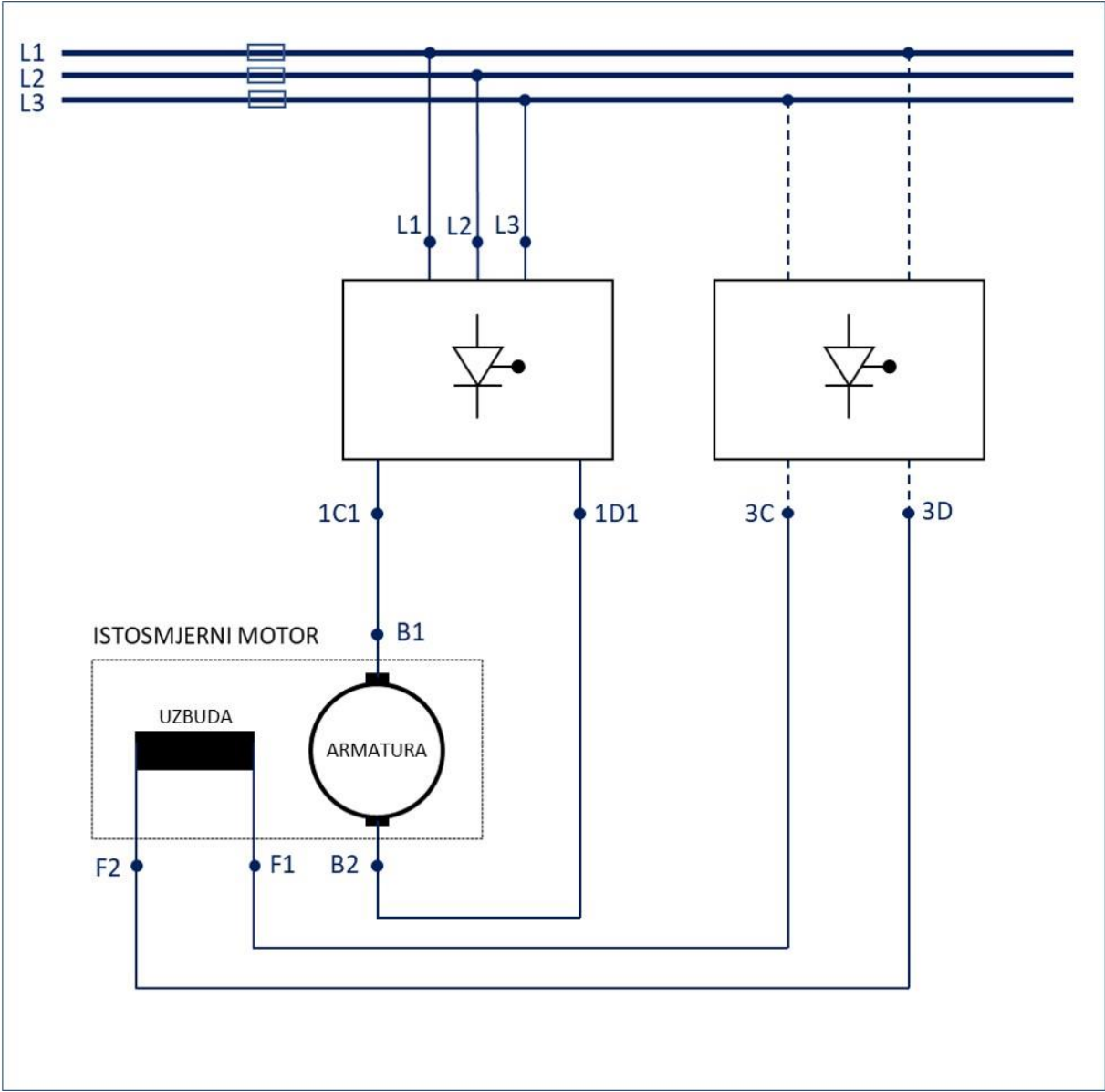
Slika 49. Shema spoja
