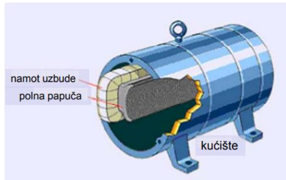
Slika 1. Stator istosmjernog stroja [2]
