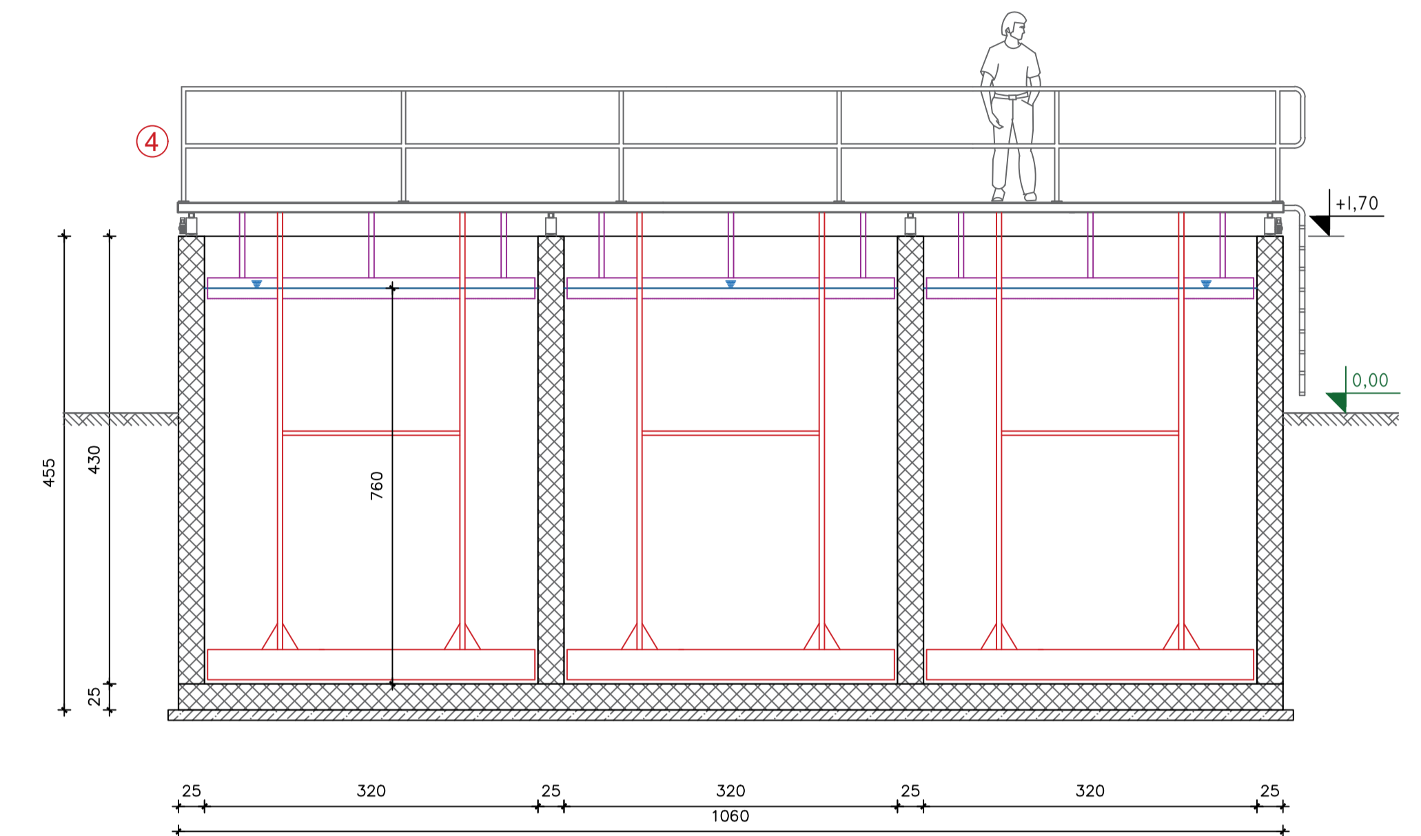
PRESJEK a-a
