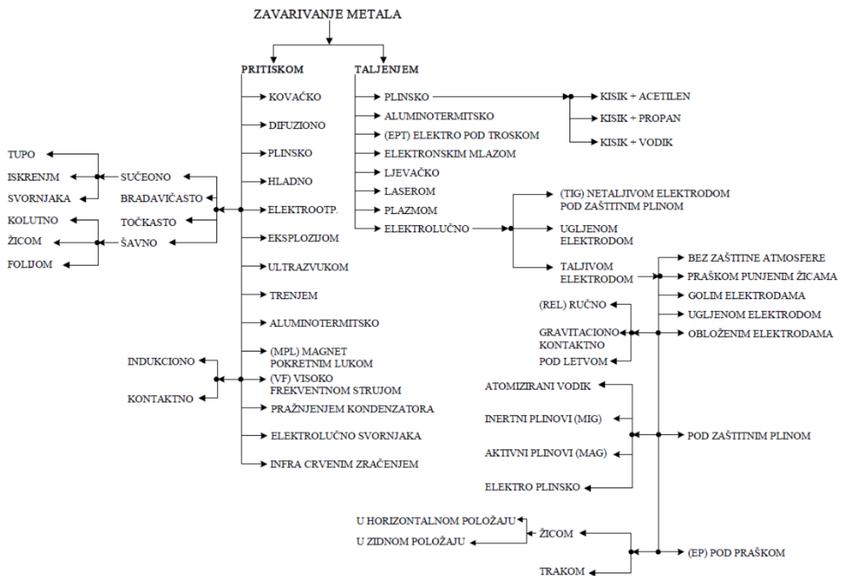
Slika 1 Prikaz svih postupaka zavarivanja [1]
