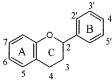
Slika 7: Struktura flavonoida
