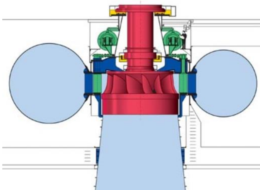
Slika 3.6. Francisova turbina [19]
