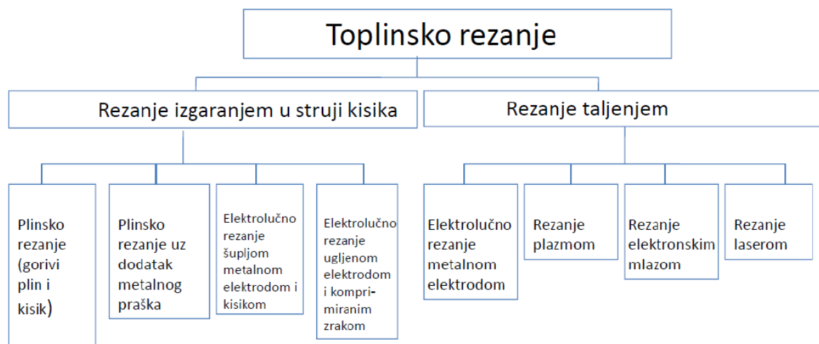
Slika 1. Podjela toplinskih postupaka rezanja [1]
