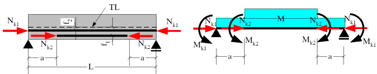
Slika 3.4. Nosac 4
