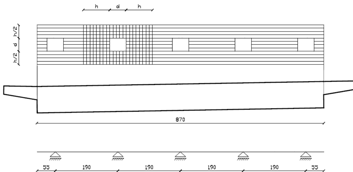
Slika 4.11 Model skrivene grede (Izvor: Autor)
