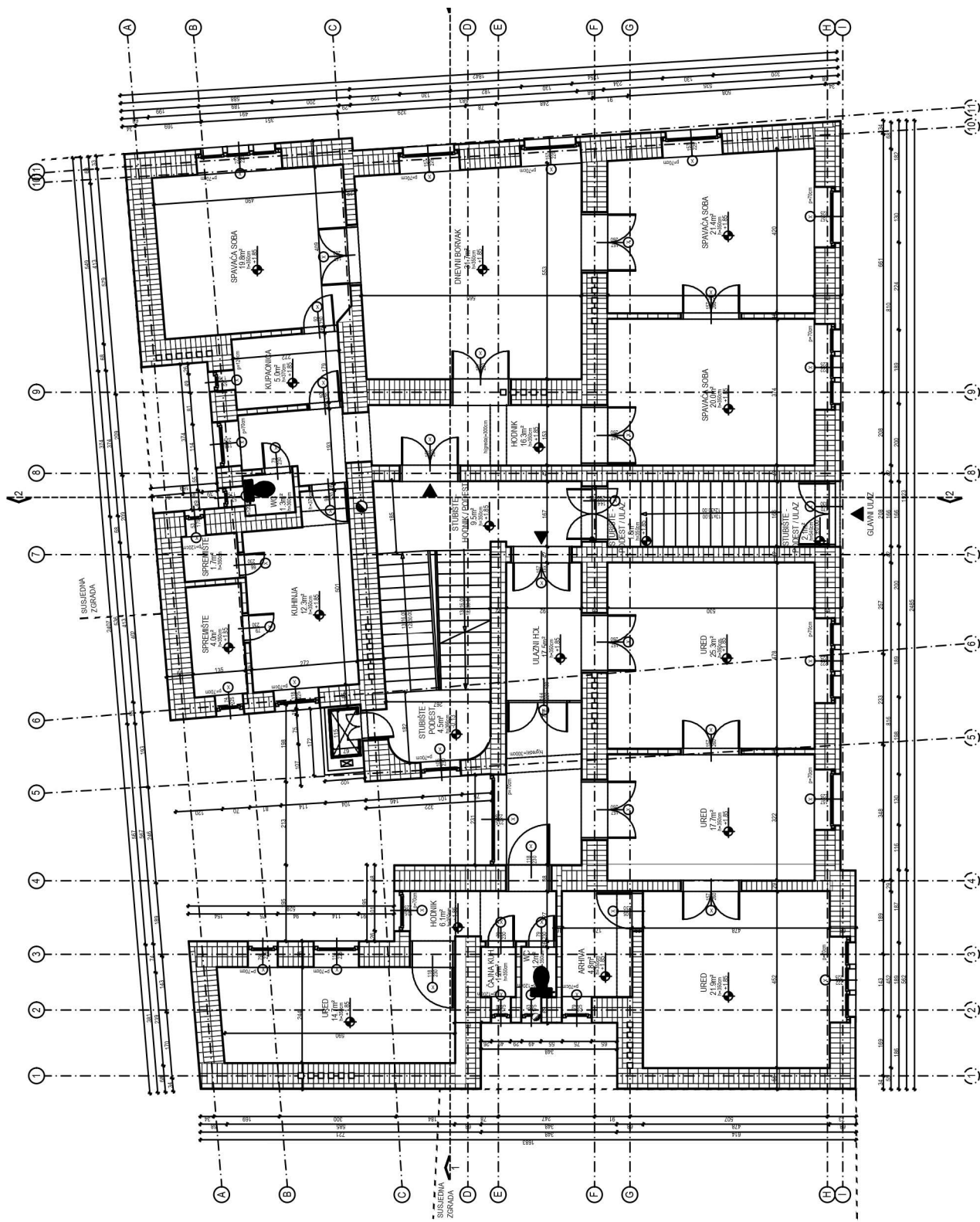
Slika 2.7 Prikaz tlocrt prizemlja
