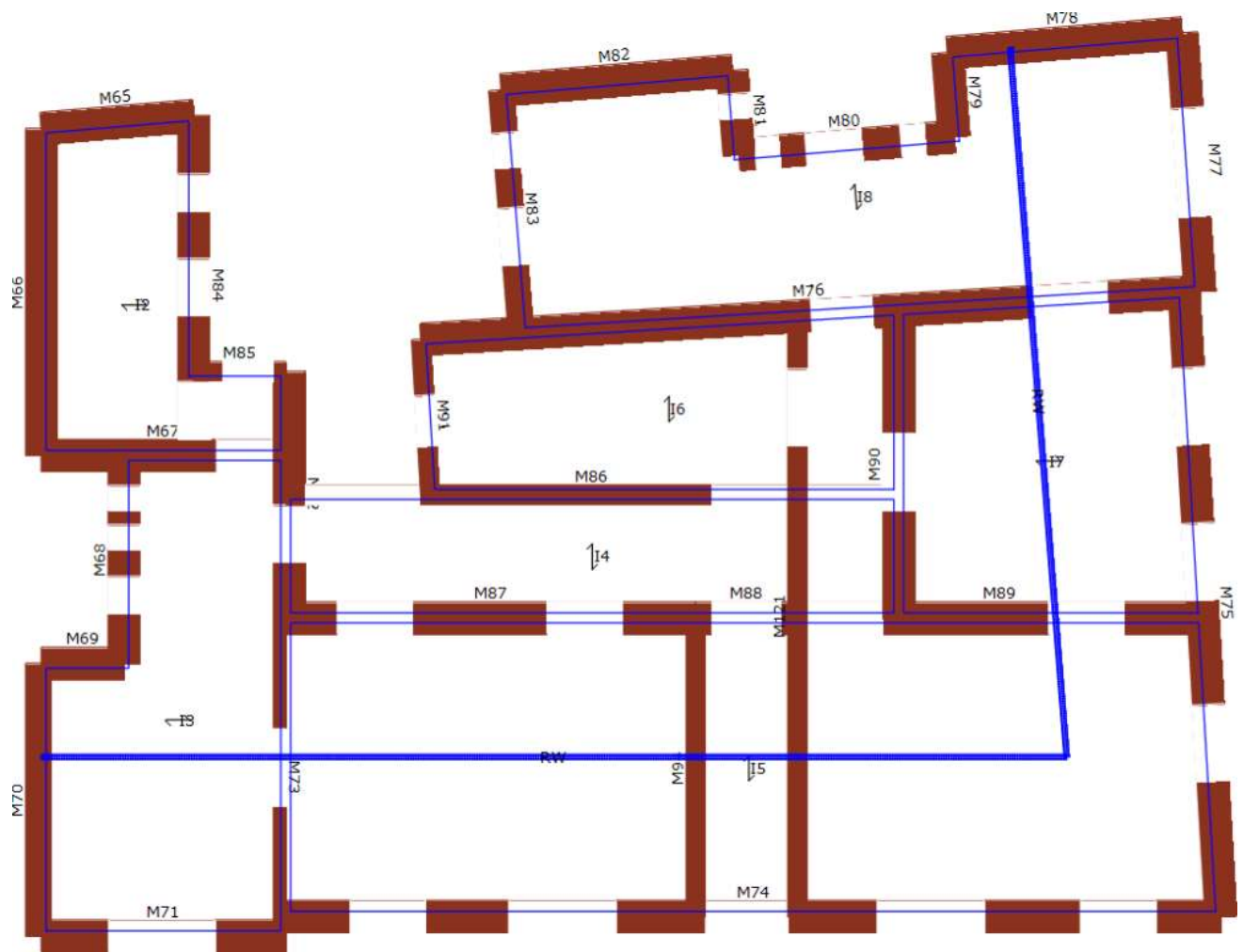
Slika 3.2 Tlocrtni prikaz etaže 2
