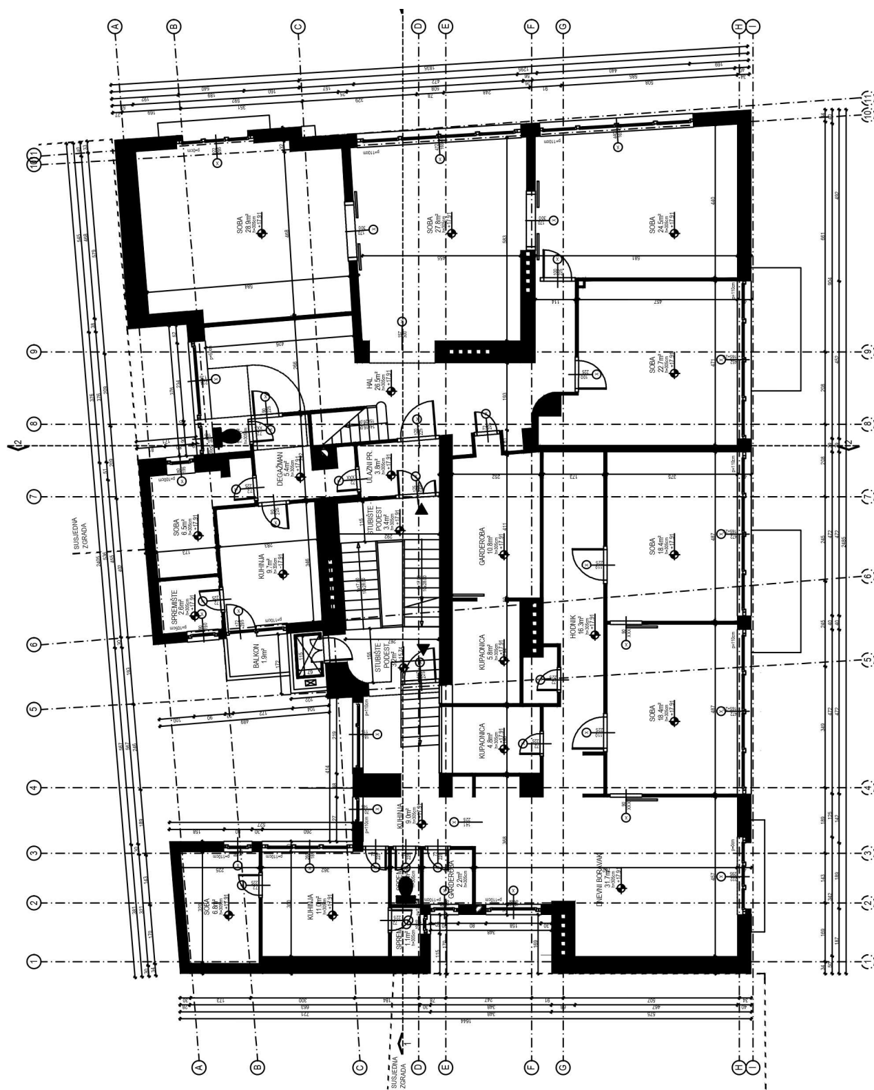
Slika 2.11 Prikaz tlocrta 4. katu
