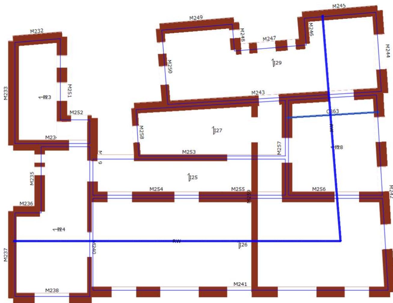
Slika 3.5 Tlocrtni prikaz etaže 5
