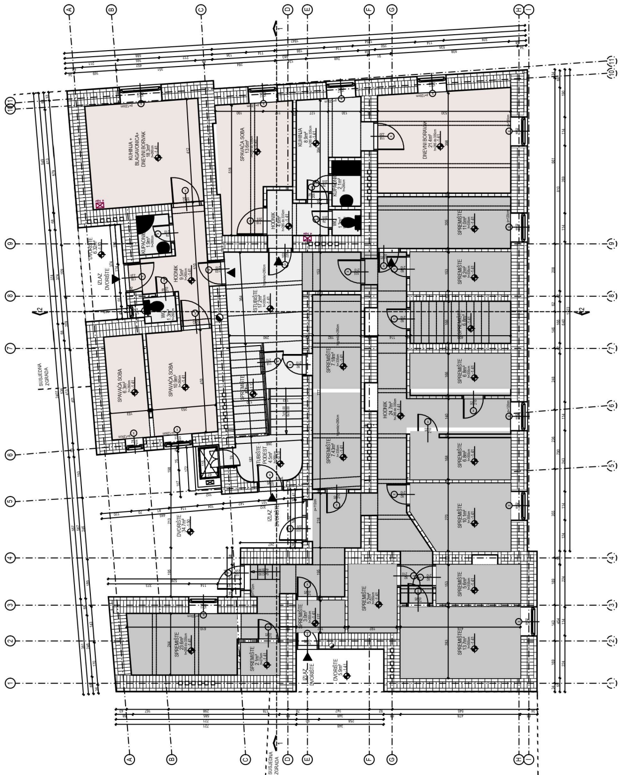
Slika 2.6 Prikaz tlocrta suterena
