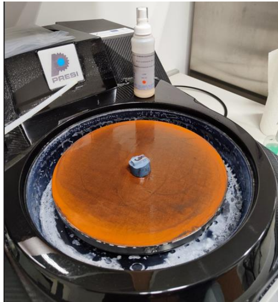
Slika 41 - Poliranje s 9 \mu m
