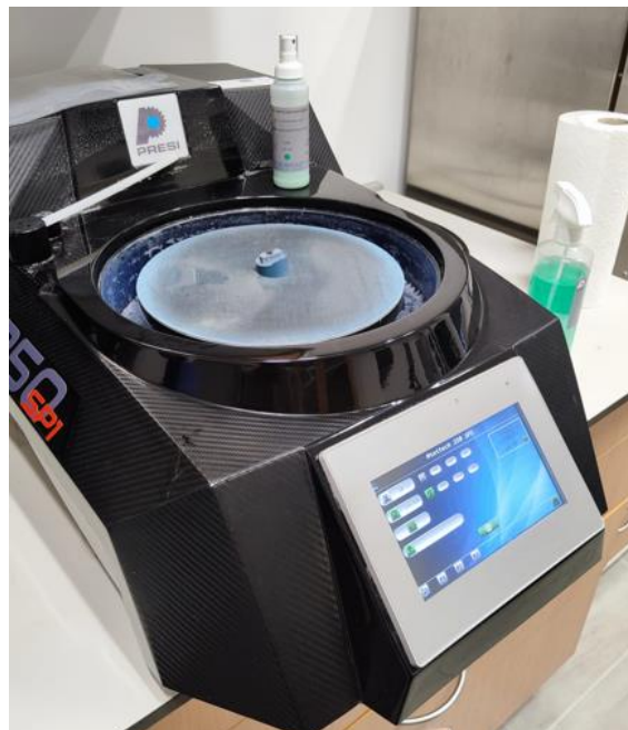
Slika 42 - Poliranje s 3 \mu m
