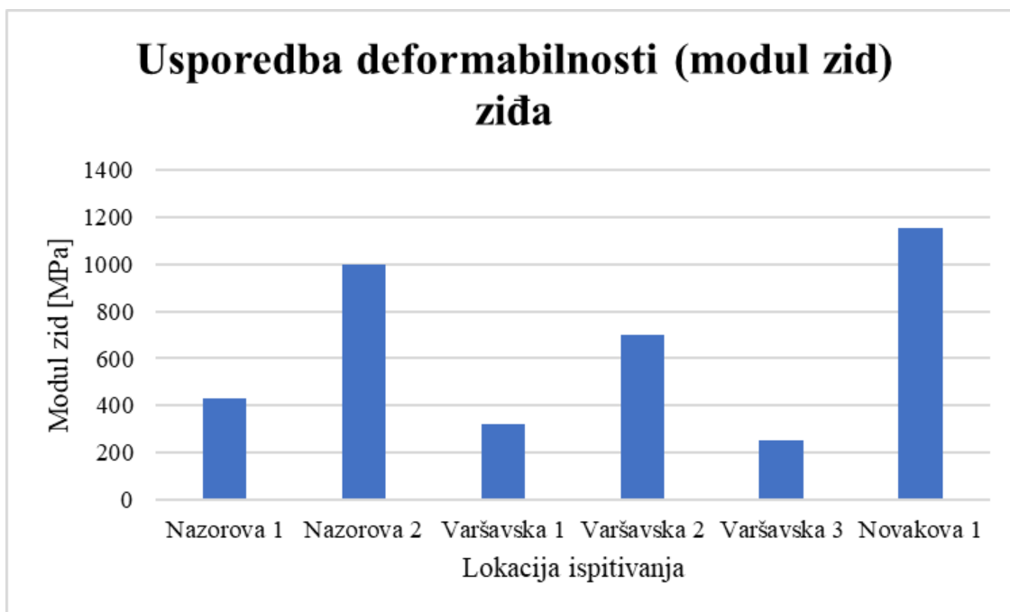
Slika 67. Grafički prikaz usporedbe deformabilnosti zida
