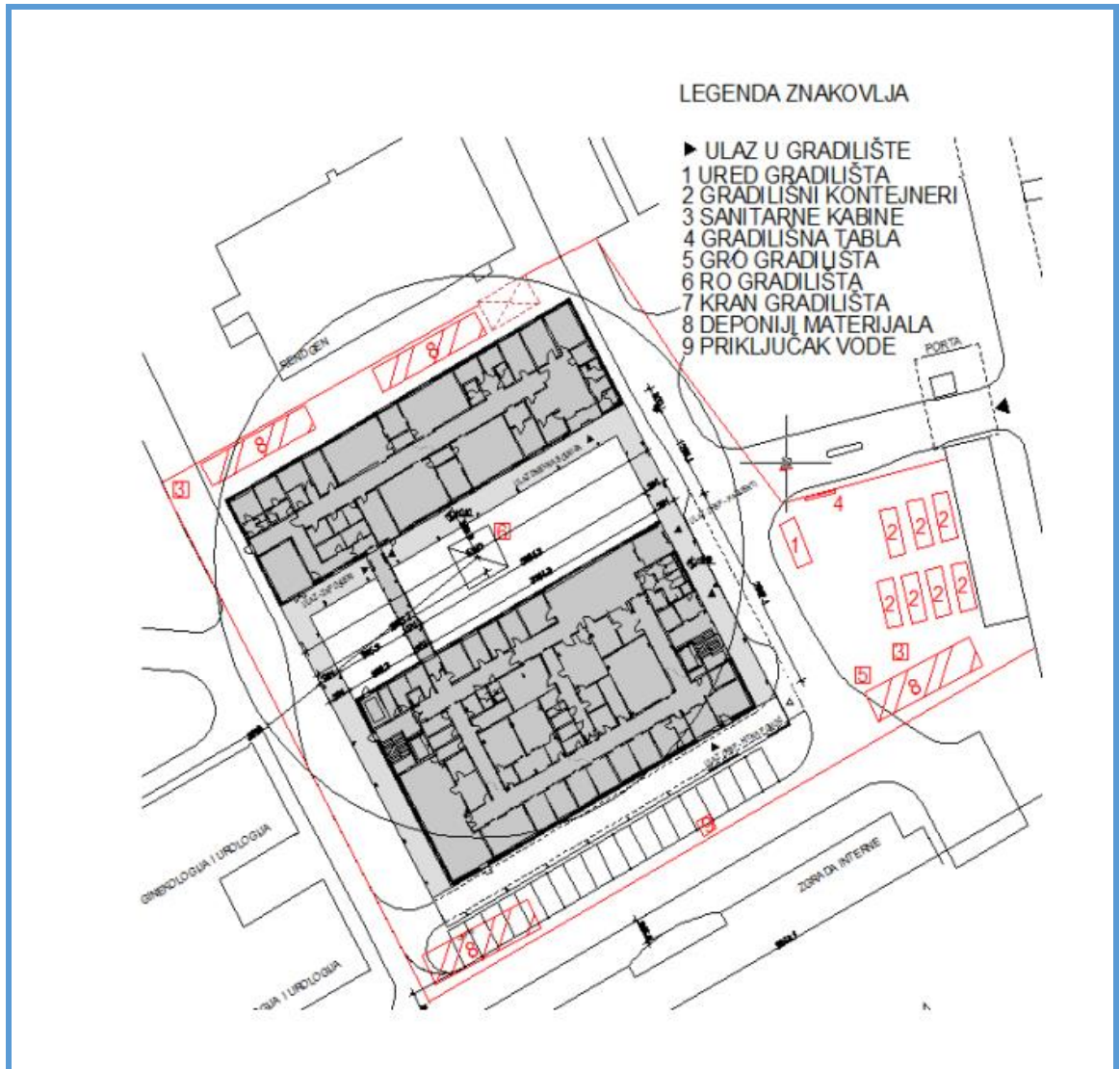
Slika 58. Shema gradilišta [11]
