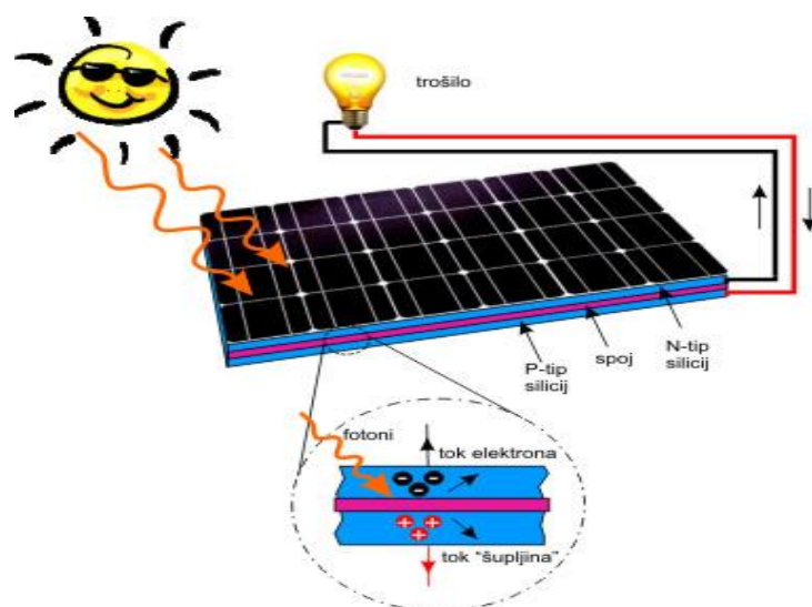
Slika 2.10. FOTONAPONSKI EFEKT [16]
