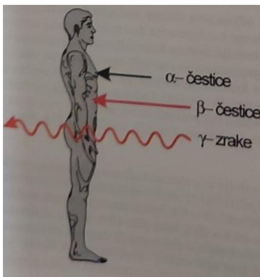
Slika 3: Prodornost pojedinih vrsta radioaktivnog zračenja [10]
