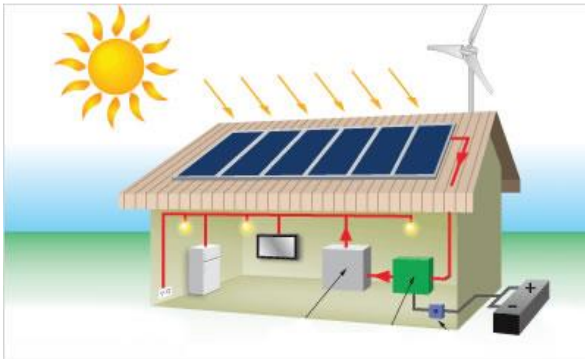
Slika 2. Off-grid sustav [3].
