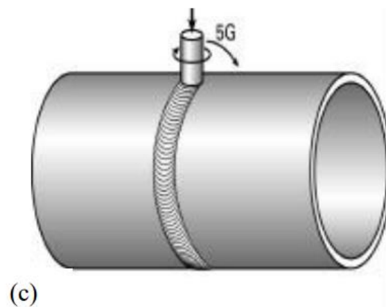
Slika 3.22 Primjer pozicijskog zavarivanja trenjem rotirajućim alatom: a) zavarivanje šupljeg elementa, b) zavarivanje šupljeg elementa, c) zavarivanje nepomične horizontalne cijevi [15]
