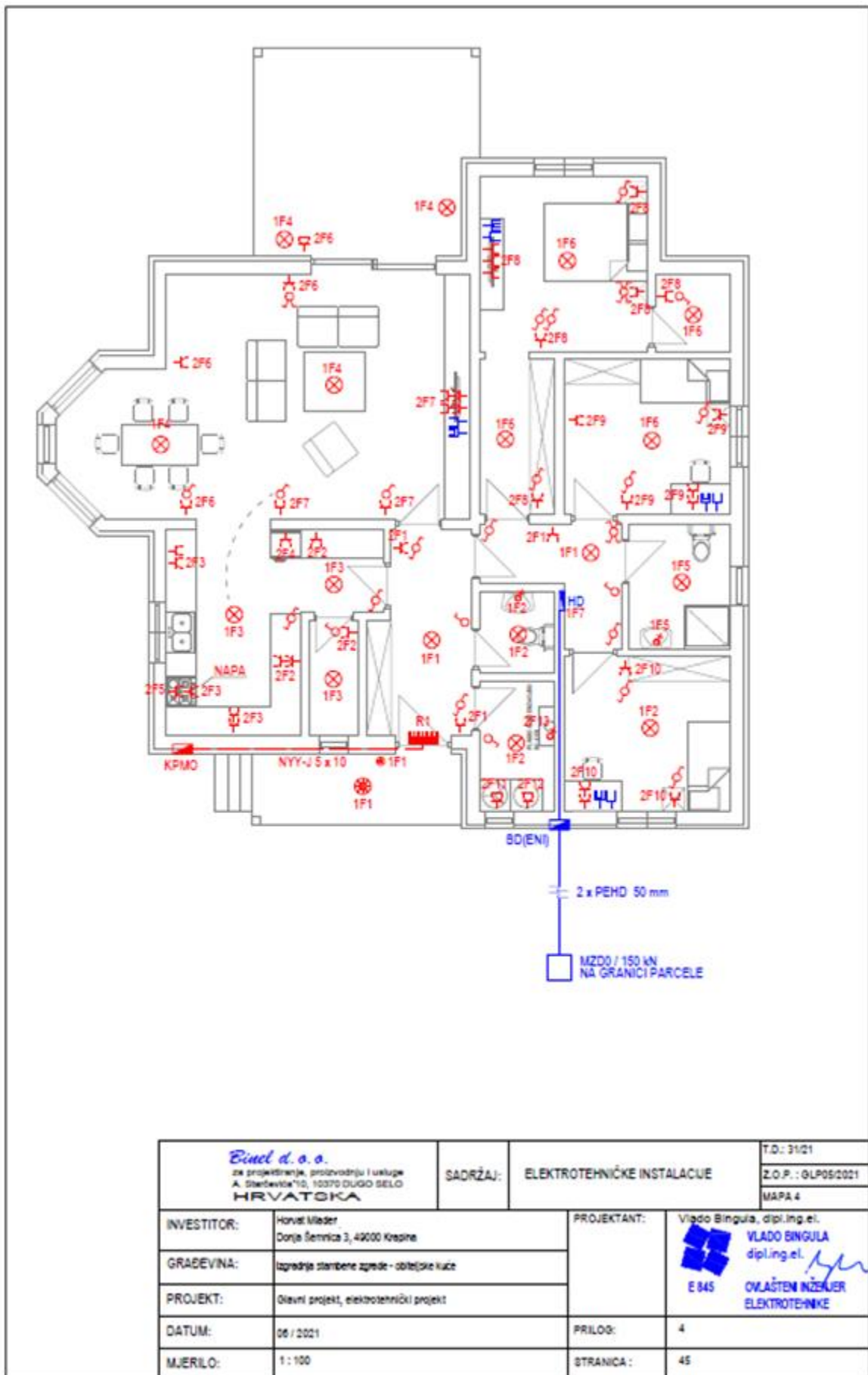
Slika 5. Projekt električne instalacije [3]
