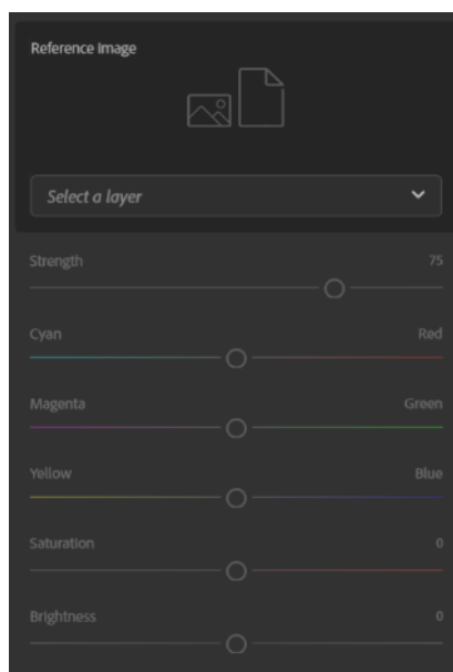
Slika 9: Harmonization : Sučelje
