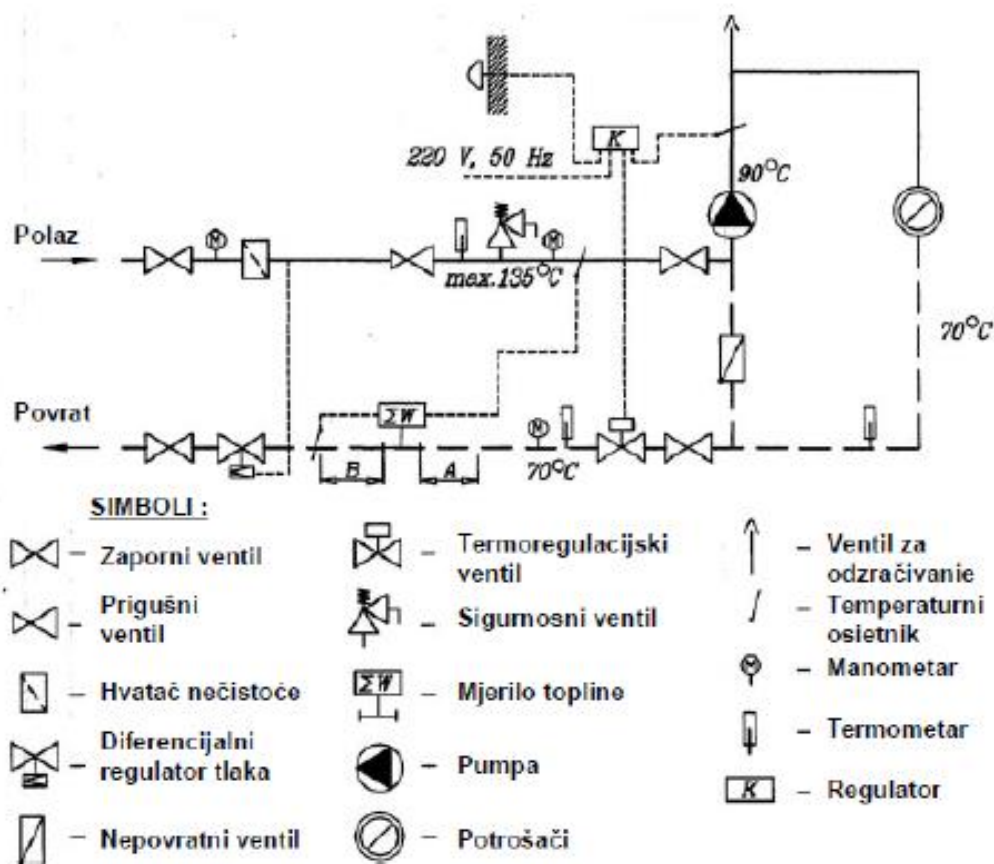
Slika 3.3.1.1; Indirektan priključak[12]
