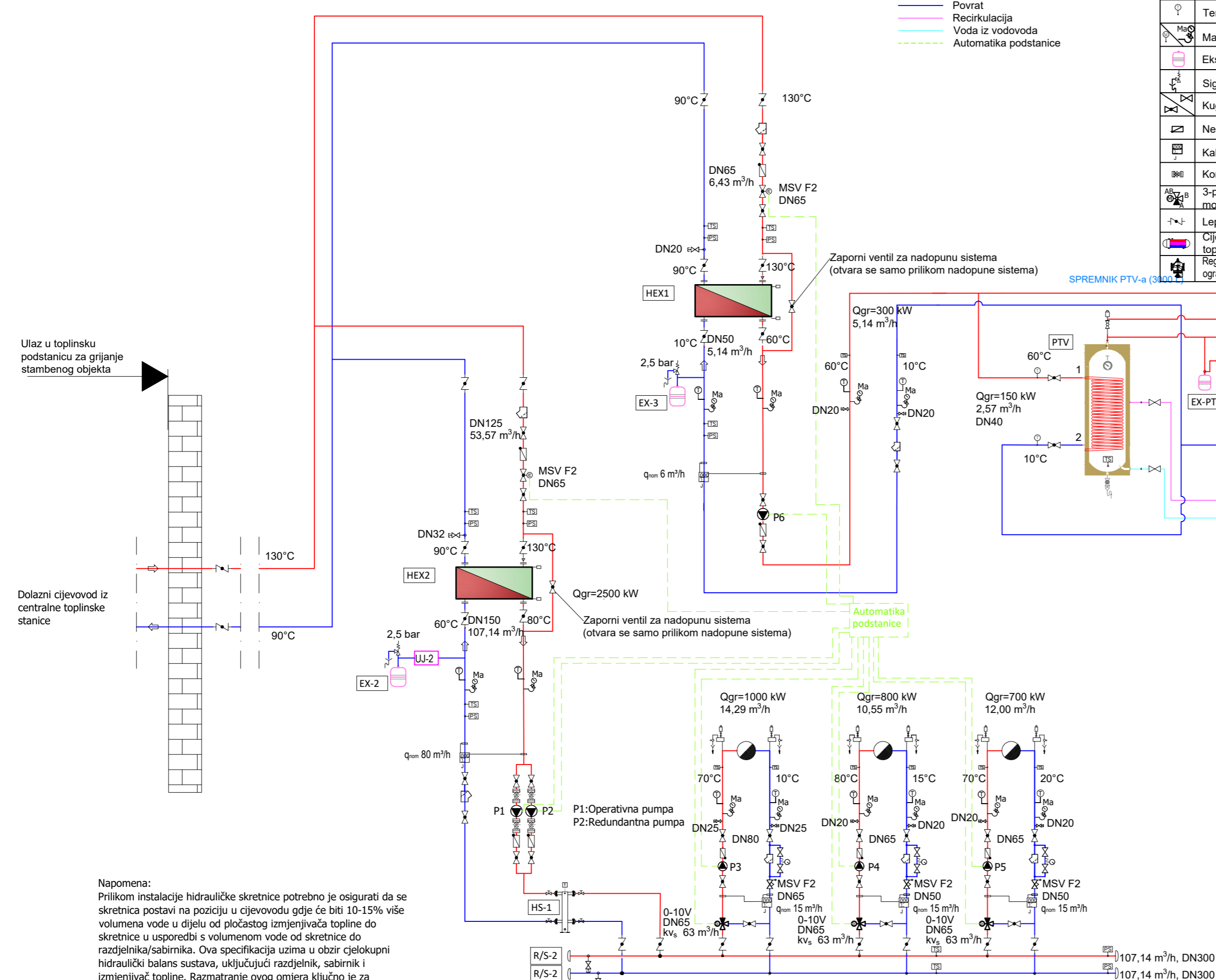
Prilog br. 21 Hidraulička shema indirektnog sustava grijanja i PTV-a (pločasti izmjenjivač) [autor]
