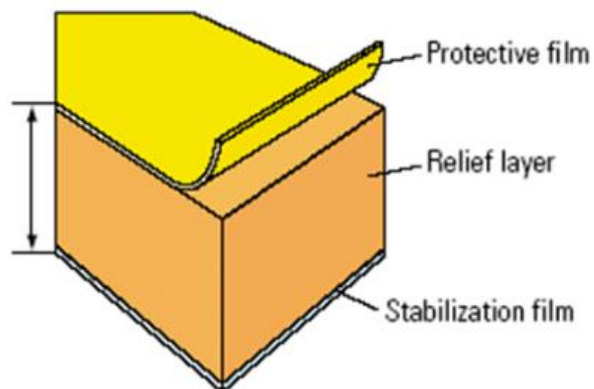
Slika 1 Građa tiskovne forme (Materijali s predavanja)
