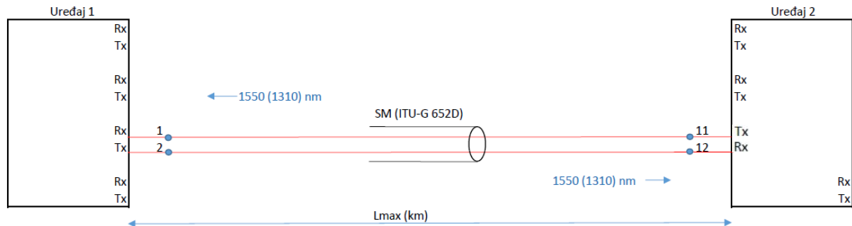
Slika 2.7. Konfiguracija spojne mreže sa aktivnim uređajima (izvor: autor)
