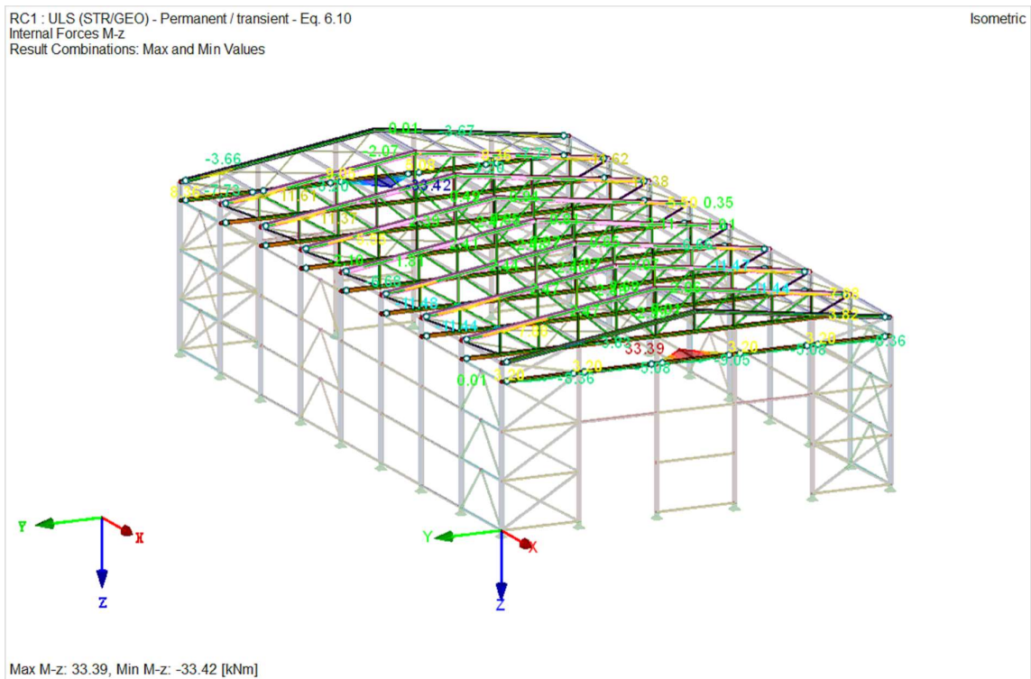
Slika 4.5.10.: Momenti savijanja u smjeru z u rešetki
