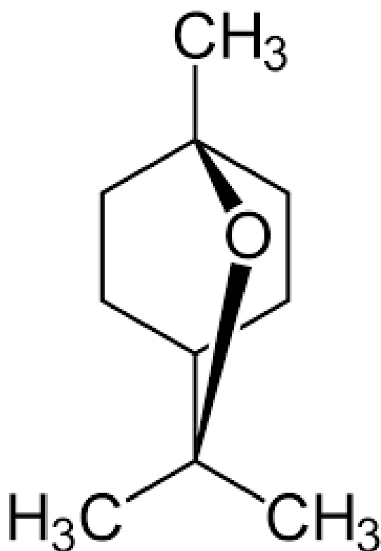
Slika 15. 1,8 – cineol
