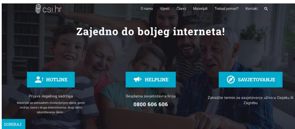
Slika 11 CSI pomoć
