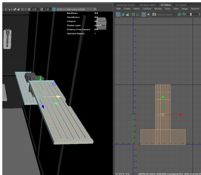
Slika 56 – „UV editor“
