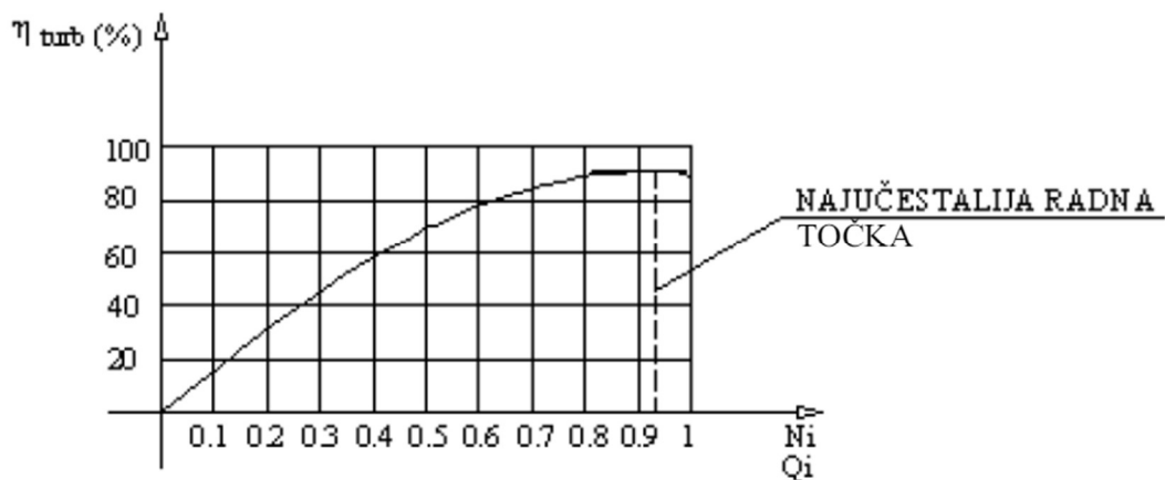
Slika 4. Učinkovitost turbine [2]
