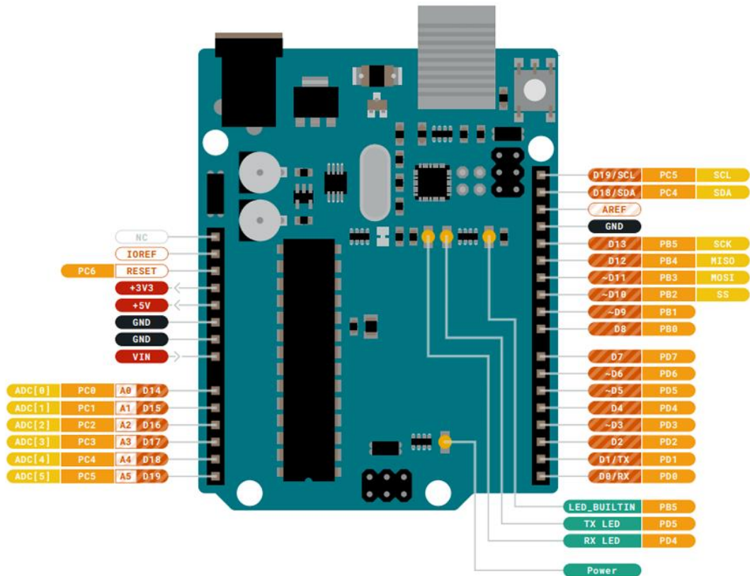
Slika 2.9. - Konektor pin-ovi Arduino Uno-a Rev3 [10]
