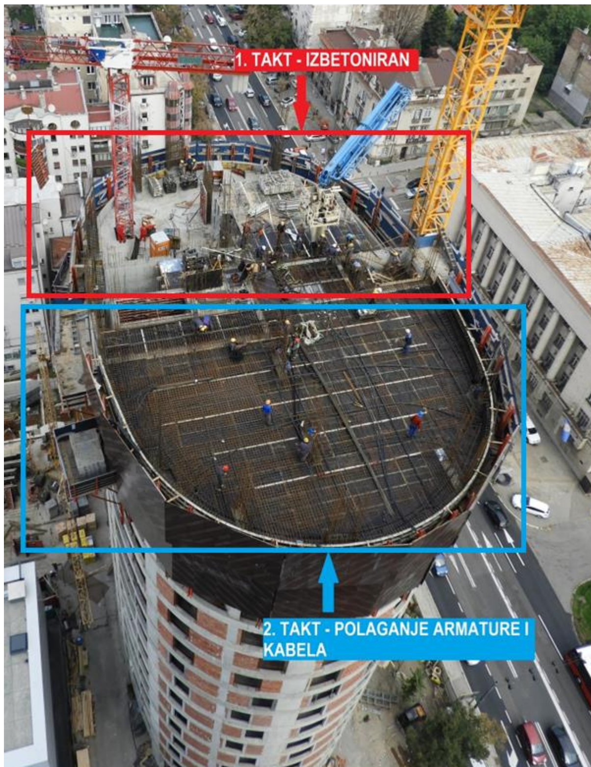
Slika 3.11 Izgradnja karakteristične ploče – prikaz dvaju taktova (Izvor: [4])
