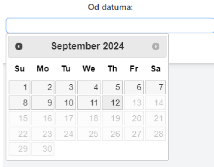
Slika 28: Datepicker
