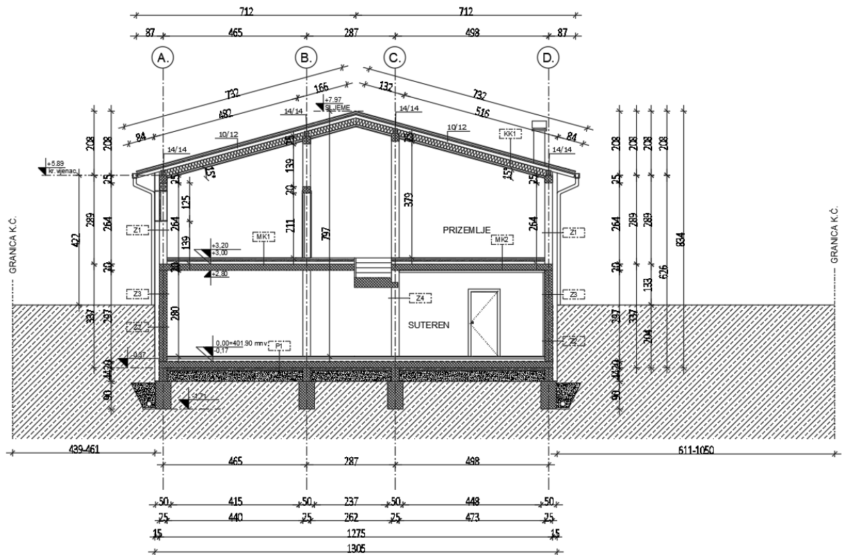
Slika 2.3 Presjek - M 1:100
