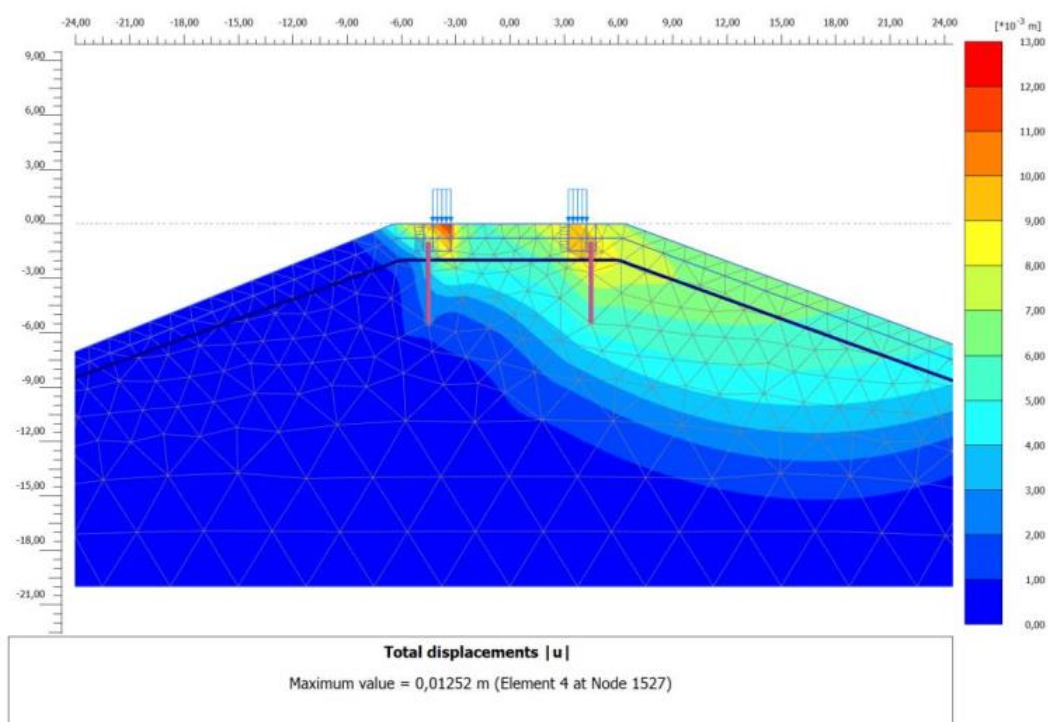
Slika 43: Prikaz ukupnog pomaka sa izvedenim pilotima od djelovanja potresnog opterećenja [7]
