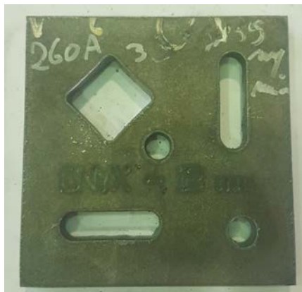
Slika 4.3.36. Uzorak B7.3 debljine 12 mm s podacima o rezanju
