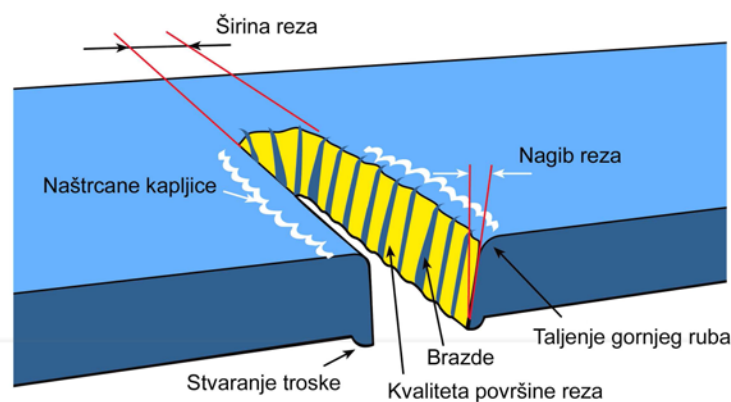
Slika 3.5. a) Izgled plazma reza sa svim parametrima [2]
