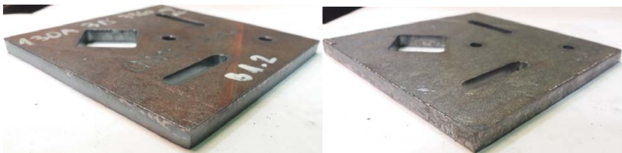
Slika 4.3.27. Uzorak B5.2 debljine 8 mm slikan s gornje i donje strane
