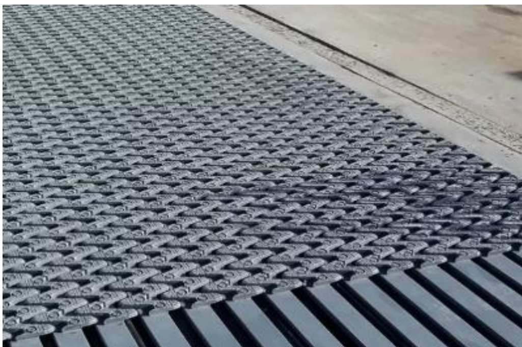
Slika 29 Modularna prijelazna naprava, [4]
