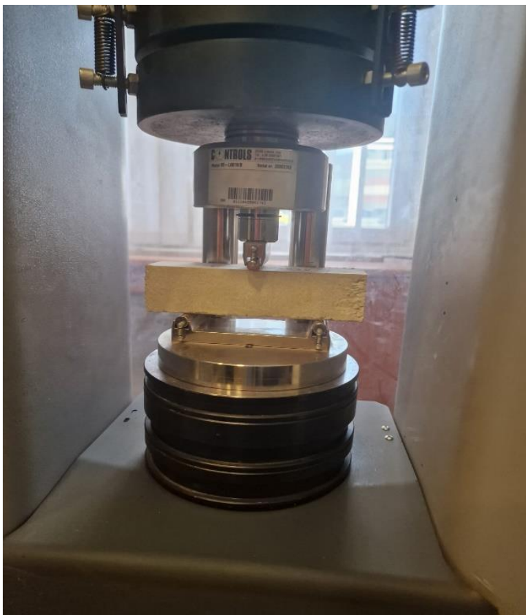
Slika 54. Ispitivanje vlačne čvrstoće
