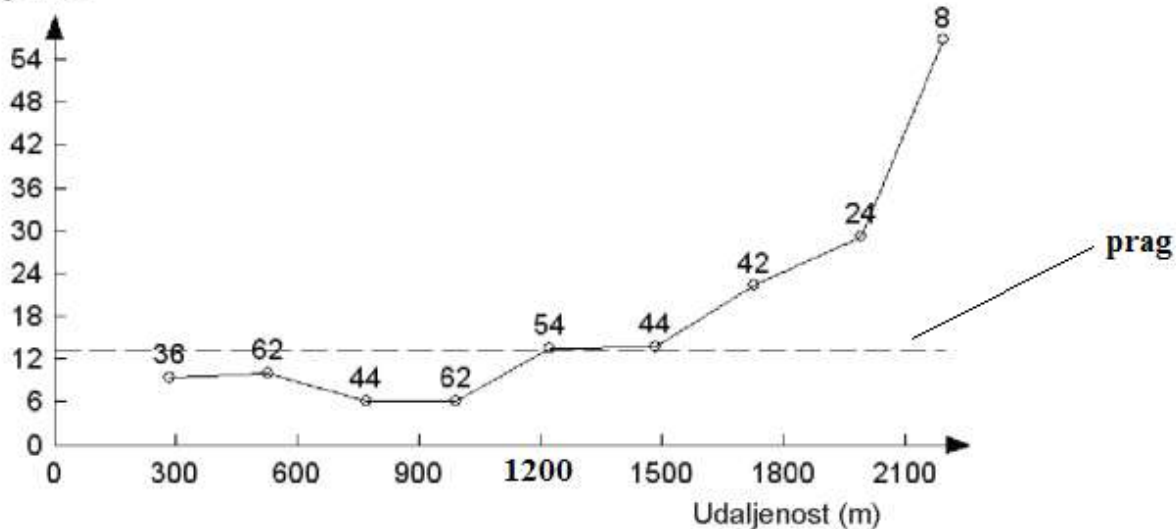
Slika 2.2.1 Neusmjereni variogram
