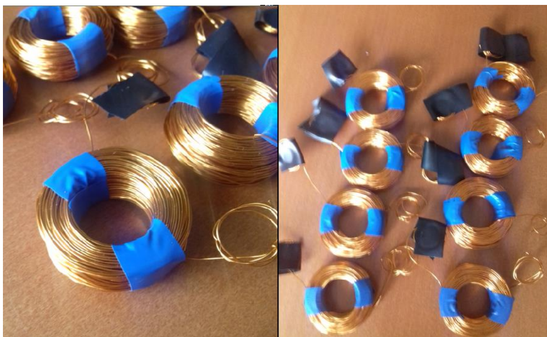
Slika 28: Gotovi namotaji
