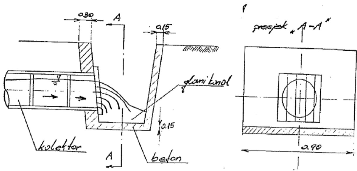
Slika 5.3 Glavni kolektor - presjek
