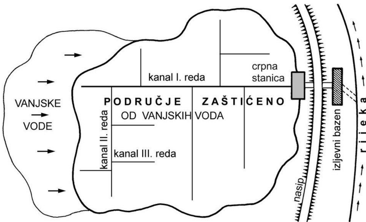
Slika 2.1 Mreža hidromelioracijskog sustava odvodnje
