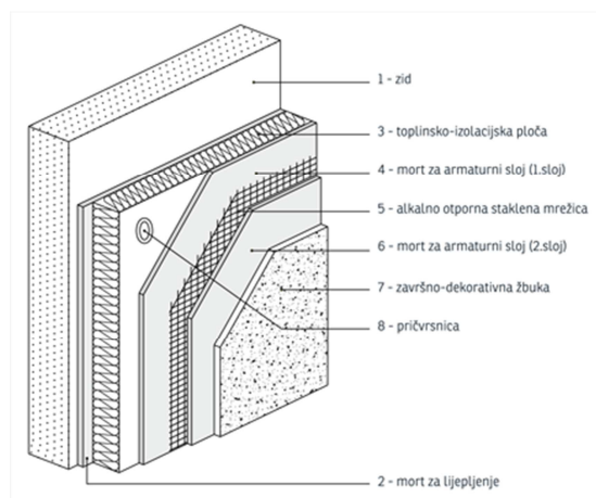
Slika 2.11 ETICS sustav
